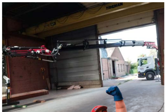
MANUTENTION GRUE À L'HORIZONTALE
